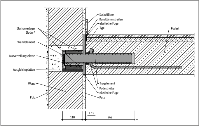
Abb. 13: Schöck Tronsole® Typ P: mit Ortbetondeckel und Tronsole® Typ L
