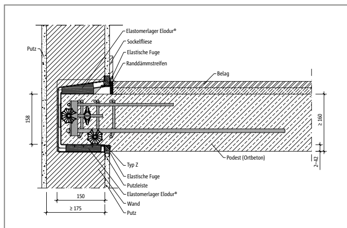
Abb. 15: Schöck Tronsole® Typ Z-V+V-T: Einbausschnitt Ort betonpodest
