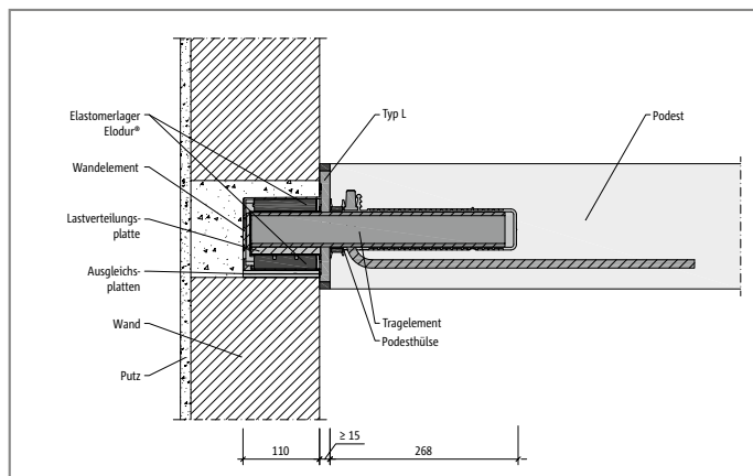
Abb. 11: Schöck Tronsole® Typ P: Einbauschnitt mit Fertigteilpodest und Tronsole® Typ L
