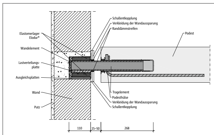
Abb. 12: Schöck Tronsole® Typ P: Einbauschnitt mit Fertigteilpodest und Luftfuge
