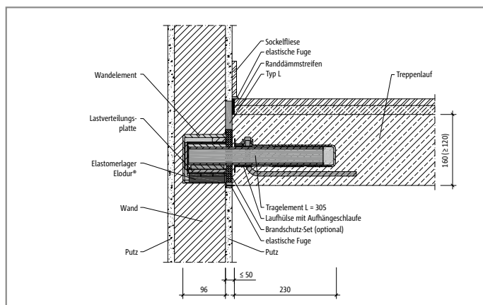
Abb. 17: Schöck Tronsole® Typ Q-FV oder Q-A2: Einbauschnitt Wanddicke 11,5 cm
