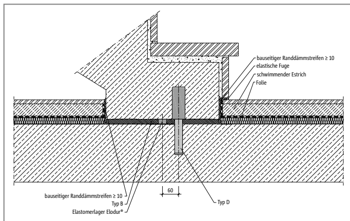
Abb. 24: Schöck Tronsole® Typ B + Typ D: Einbausschnitt
