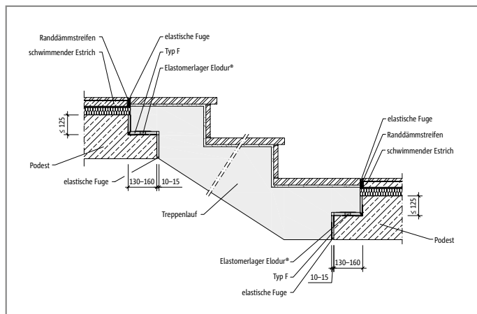
Abb. 22: Schöck Tronsole® Typ F: Einbauschchnitt
