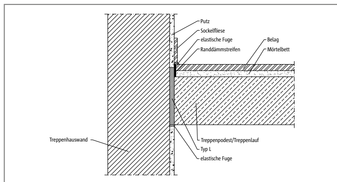
Abb. 27: Schöck Tronsole® Typ L: Einbauschnitt Ortbetontreppe
