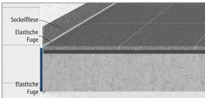
Abb. 32: Sockelfliese und Belag mit elastischer Fuge trennen
