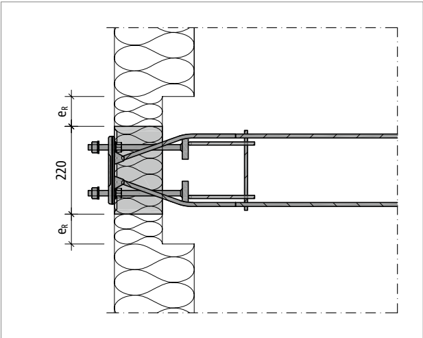
Abb. 86: Schöck Isokorb® XT Typ SQ: Randabstände
