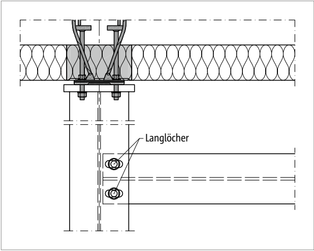
Abb. 85: Schöck Isokorb® XT Typ SQ: Dehnfugendetail zur Ermöglichung der Verschieblichkeit bei Temperaturdehnung
