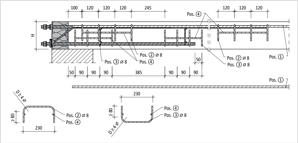
Abb. 55: Schöck Isokorb® XT Typ SK-MM2: Bauseitige Bewehrung mit Bügel Ø 8 mm; Schnitt
