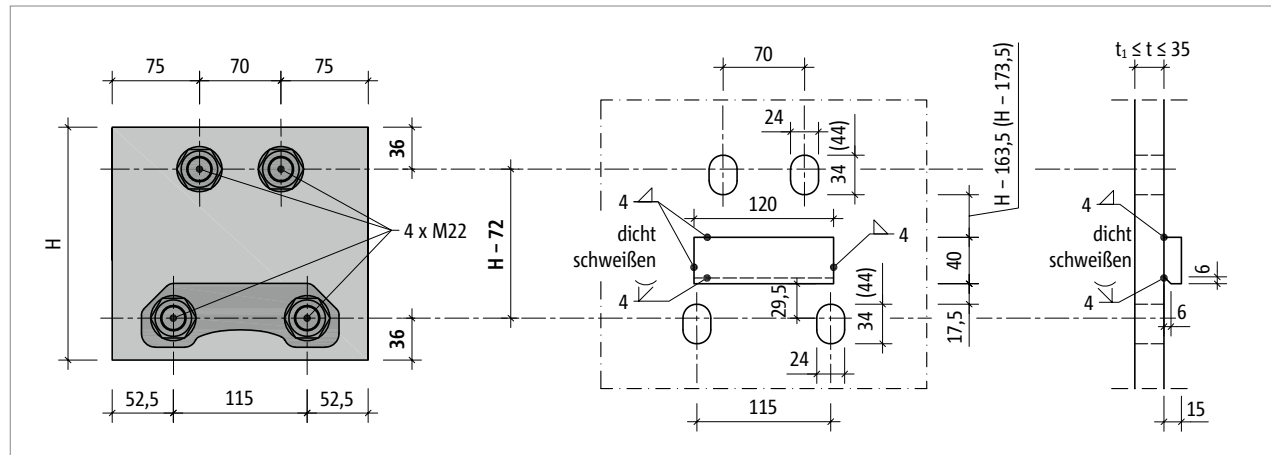
Abb. 67: Schöck Isokorb® XT Typ SK-MM2 mit CV26: Konstruktion des Stirnplattenanschlusses mit Betondeckung CV26 (ersetzt durch XT Typ SK-MM2....-CV28)
