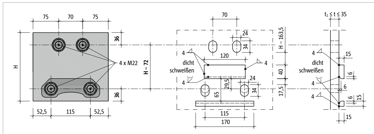
Abb. 68: Schöck Isokorb® XT Typ SK-MM2 mit CV26: Konstruktion des Stirnplattenanschlusses mit Betondeckung CV26; Rundlöcher unten, alternativ Langlöcher und eine zweite Knappe zur Übertragung der negativen Querkraft (ersetzt durch XT Typ SK-MM2....-CV28)
