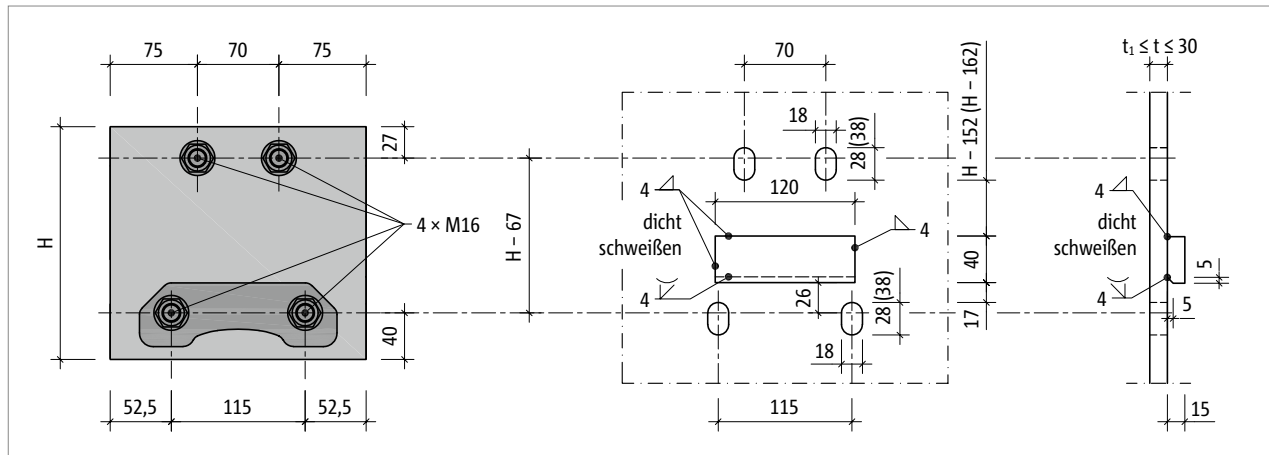
Abb. 63: Schöck Isokorb® XT Typ SK-M1: Konstruktion des Stirnplattenanschlusses
