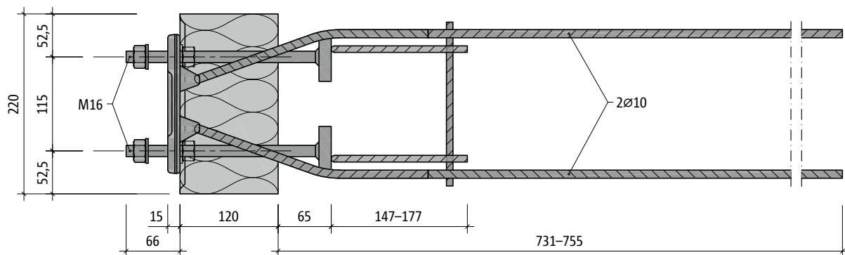
Abb. 90: Schöck Isokorb® XT Typ SQ-V2: Grundriss
