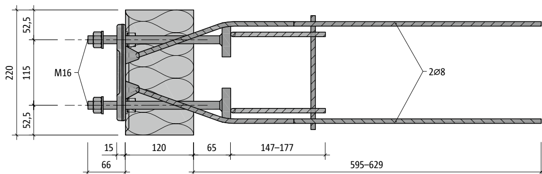
Abb. 89: Schöck Isokorb® XT Typ SQ-V1: Grundriss
