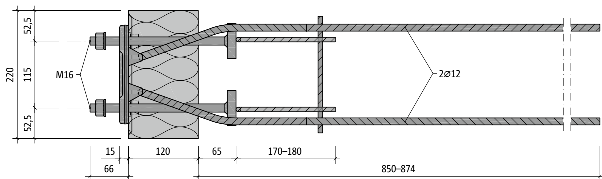
Abb. 91: Schöck Isokorb® XT Typ SQ-V3: Grundriss
