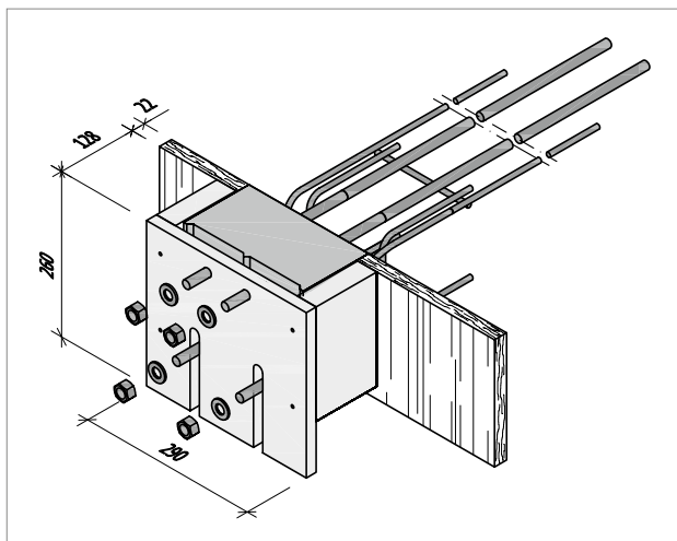
Abb. 20: Schöck Isokorb® XT Typ SK: Darstellung mit Einbauhilfe
