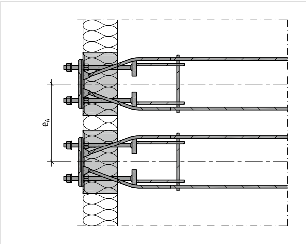
Abb. 88: Schöck Isokorb® XT Typ SQ: Achsabstand
