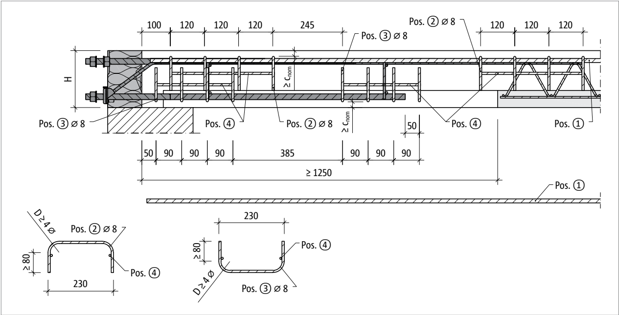
Abb. 61: Schöck Isokorb® XT Typ SK-MM2: Bauseitige Bewehrung bei Halbfertigteilbauweise mit Bügel \varnothing 8 mm; Schnitt
