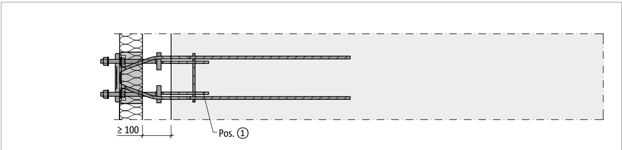
Abb. 181: Schöck Isokorb® T Typ SQ: Bauseitige Bewehrung bei Fertigteilbauweise, Grundriss
