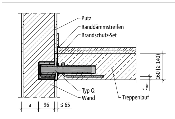
Abb. 13: Schöck Tronsole® Typ Q: Brandschutzausführung
