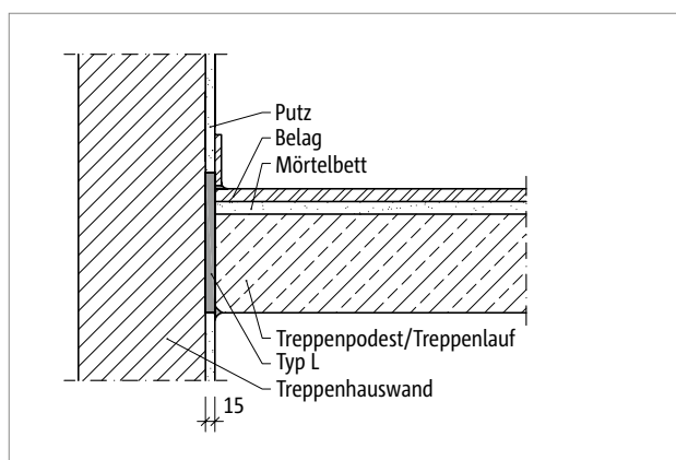
Abb. 16: Schöck Tronsole® Typ L: Brandschutzausführung
